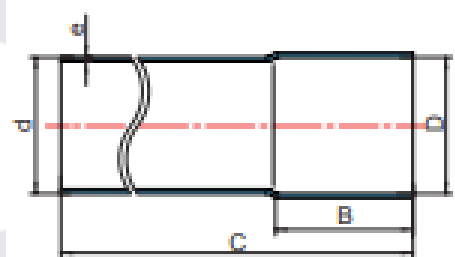
TUBO DE PVC SOLDÁVEL 3M DIMENSÕES (mm)
