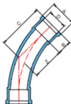
CURVA 45° SOLDÁVEL DIMENSÕES (mm)
