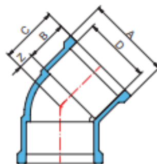
JOELHO 45° SOLDÁVEL DIMENSÕES (mm)
